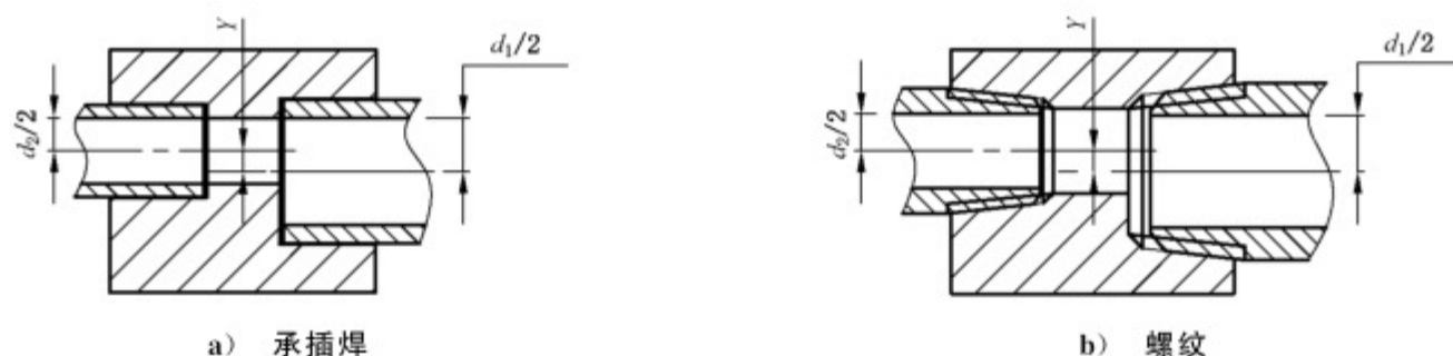
图 11 偏心异径管件的偏心距示意图
