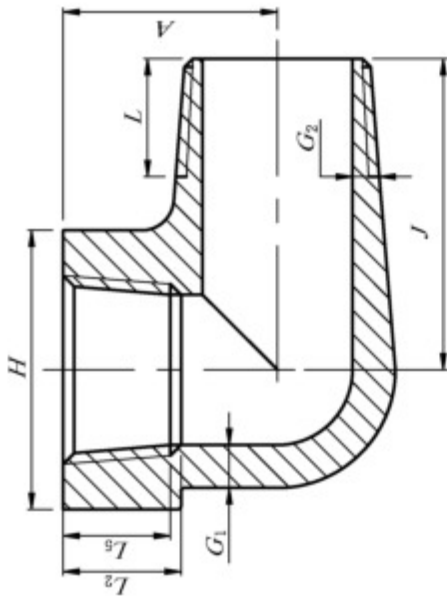
图 6 螺纹管件(内外螺纹 90°弯头/THD-90SE)形状
